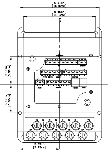
后视图
