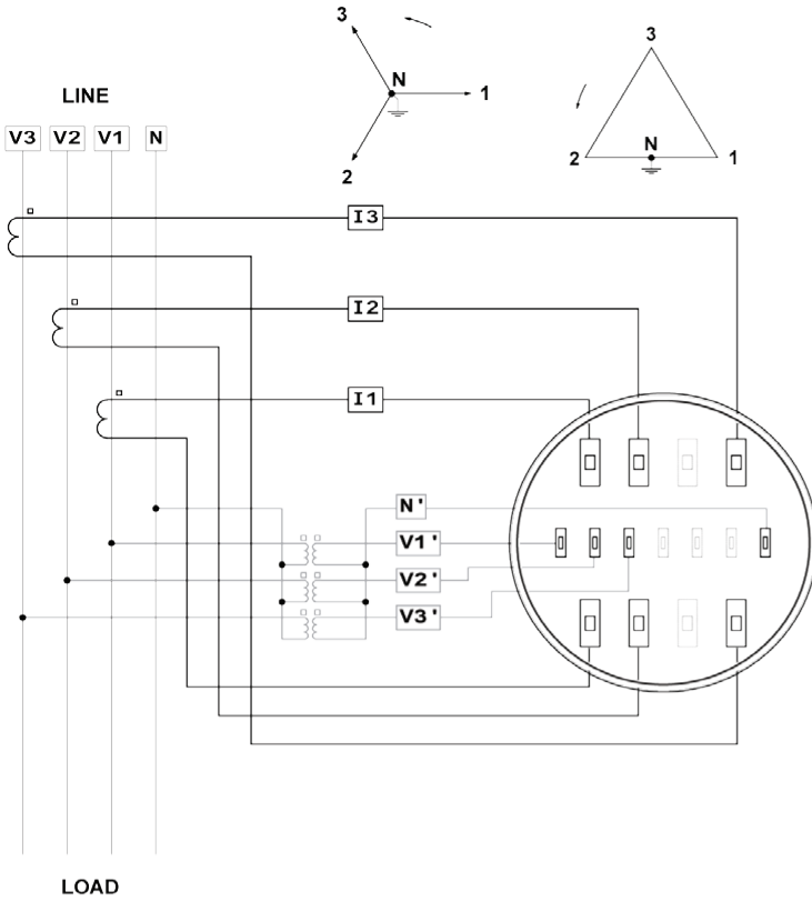
9S结构, 4线星形和三角形
