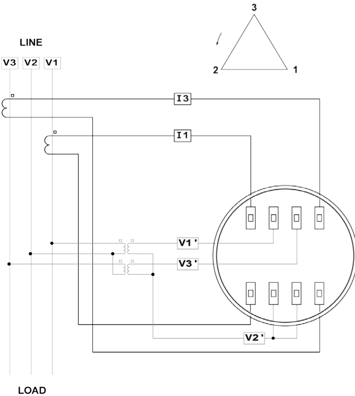
45S结构, 3线三角形
